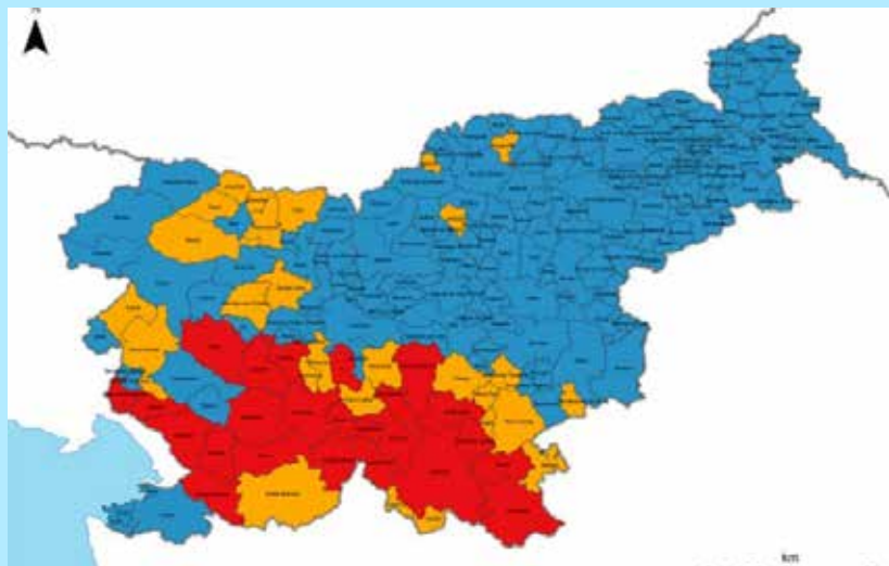
Stopnja prisotnosti radona v Sloveniji. Meritve na domu bodo izvajali predvsem v rdeče obarvanih občinah, dodatno pa tudi v oranžnih.
