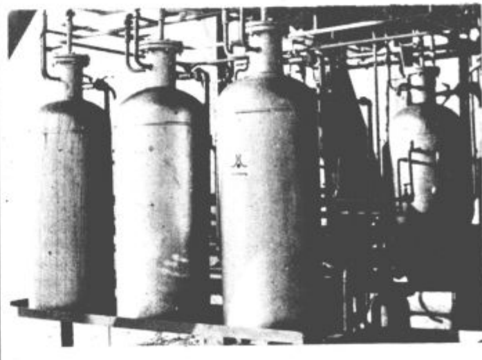
Poskusna naprava za pridobivanje bioplina
