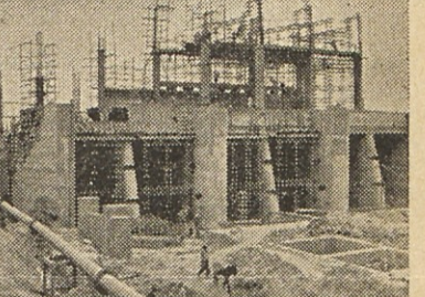
Gradišče pakistanske hidrocentrale Gujranwale. Tudi za to centralo smo dobavili tri Kaplanove agregate po pribl. 6500 KS vsak
