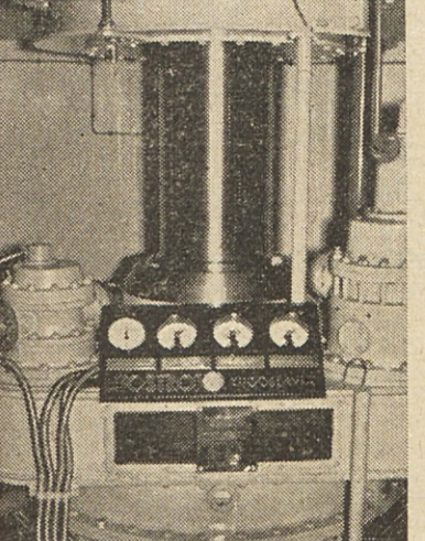
HE Chichokj Mallian — del turbinskega prostora. Za to centralo smo dobavili 3 Kaplanove turbine po 6500 KS
