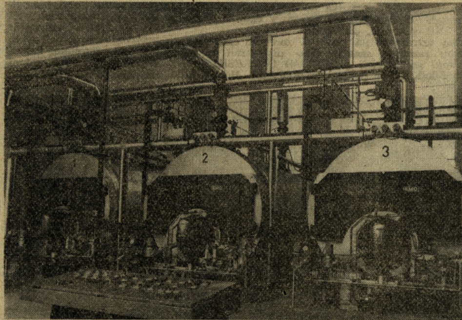
Posnetek prikazuje industrijsko kotlarnico v Iskri Kranj
