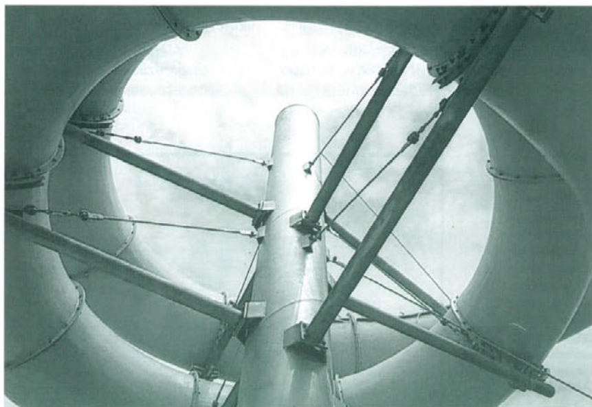
Konstrukcija vodnega tobogana v Moravskih Toplicah, delo delavcev Strojnega remonta
