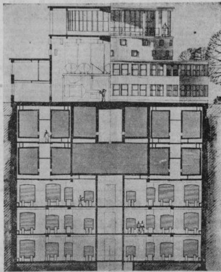
Maketa ormoške kleti nam prikazuje prerez, na katerem pride v polni meri do izraza sodobna urejenost objekta
