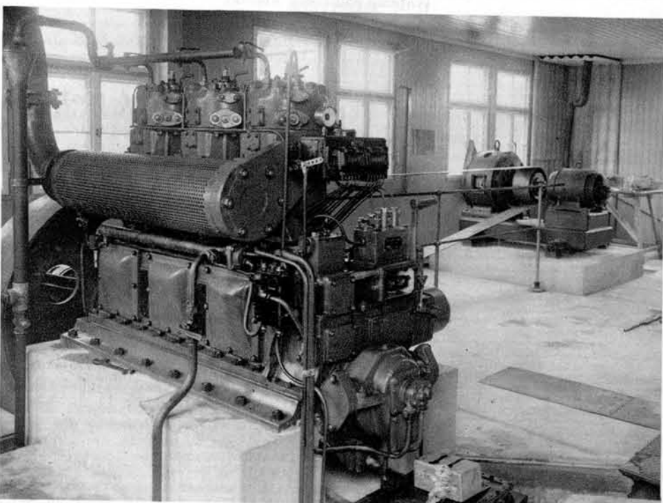
Pogonska centrala domžalske radio postaje
