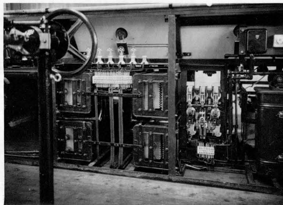
Zadnja stran stikalnega pulta
