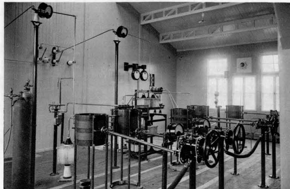
Glavna aparatura domžalske radioodajne postaje s pripravami za modulacijo in oddajo samo. Vse je zgrajeno po najmodernejših sistemih.
