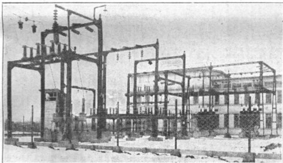
Transformatorska naprava v prosti montaži zunaj poslopja, kjer se zniža napetost velenjskega toka na 20.000 voltov.
