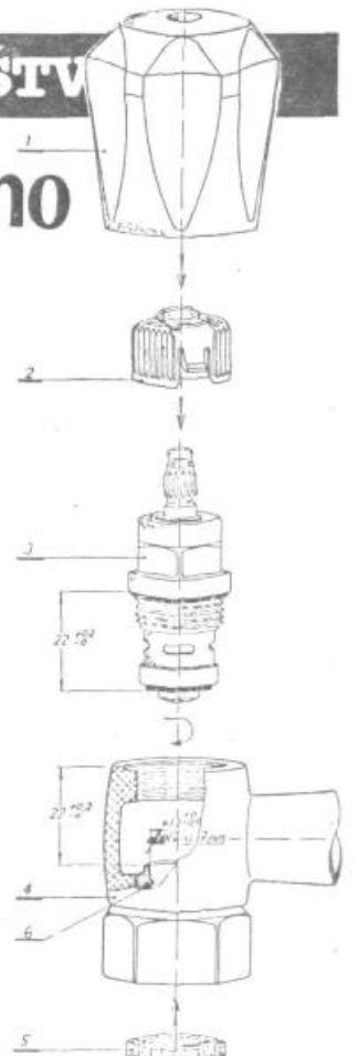
POZ.1 ROČAJ POZ.2 VMESNI ELEMENT POZ.3 BREZSUMNI VENTIL POZ.4 OHIŠJE ARMATURE POZ.5 TESNILO Z MREZO SEDEŽ POZ.6 PIPE
