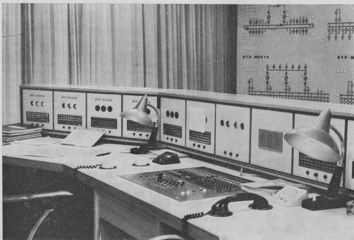
RTP Šiška 110/10 kV — razklopišče
