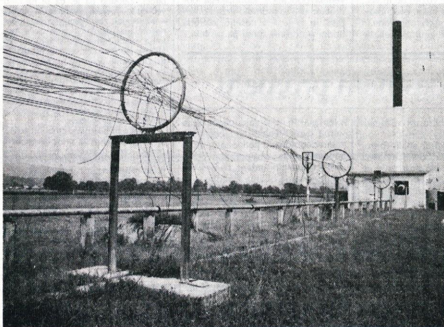
Med letalskim napadom poleti 1991 poškodovan antenski vod in antena v Domžalah
