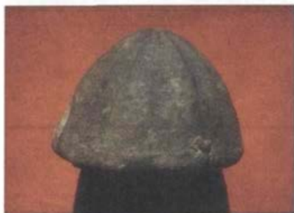
4. Fosilni morski ježek, v Istri imenovan hleb sv. Štefana. S takšnimi »kamni« naj bi kame-njali tega svetnika (foto: M. Grm).
