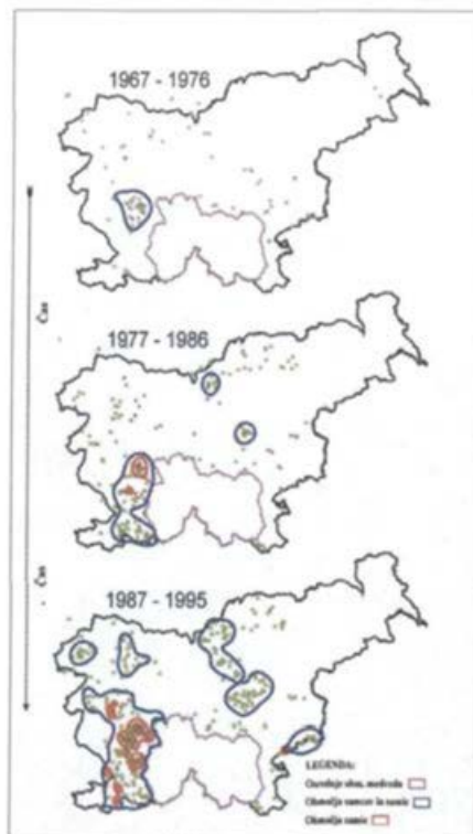
Slika 2: Prostorsko širjenje medveda iz »Osrednjega varovalnega območja« po letu 1966
