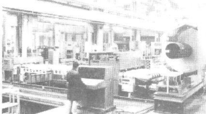
Podajna linija za avtomobilsko industrijo v ZDA, ki omogoča avtomatizirano delovanje preoblikovalnih procesov.
