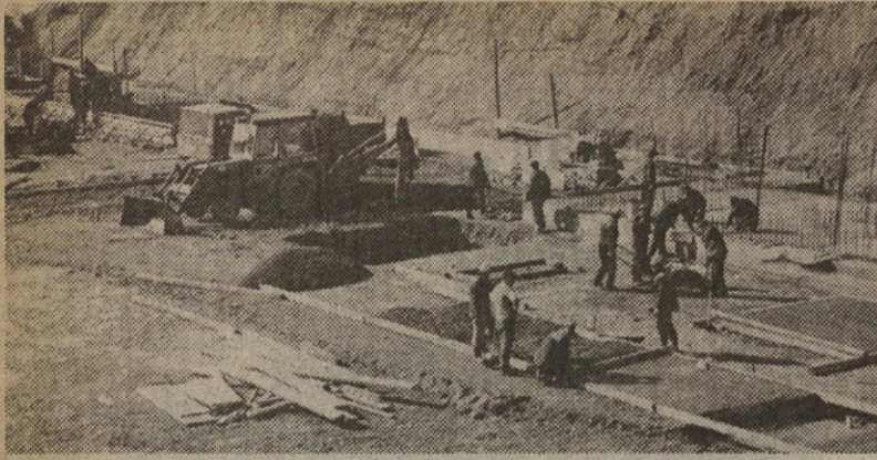
Betoniranje temeljev za stebre tistega dela stavbe, ki jo bo možno nadgraditi.
