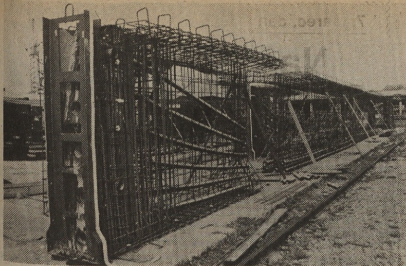
Armatura nosilcev za premostitvene objekte v Višegradu — izdelavo manjših elementov so preselili iz Maribora v Bosno
