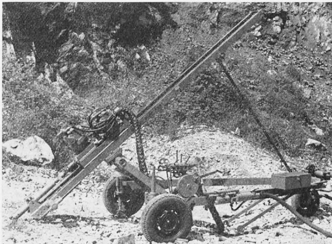
Slika 1 — pnevmatični vrtalni stroj RGVN, proizvod Zelezarne Ravne za globoke vrtnice
