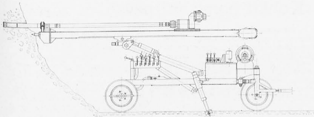
Slika 2 — pnevmatični vrtalni stroj za globoko vrtanje — kladivo RK-15 ali RK-26 v vrtini
