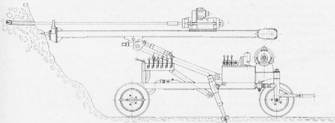
Slika 3 — pnevmatični vrtalni stroj s težkim udarno rotacijskim kladivom na lafeti
