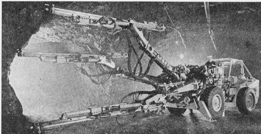
Slika 6 — pnevmatični vrtalni stroj s tremi lafetami za gradnjo predorov, kamnolomov itn.
