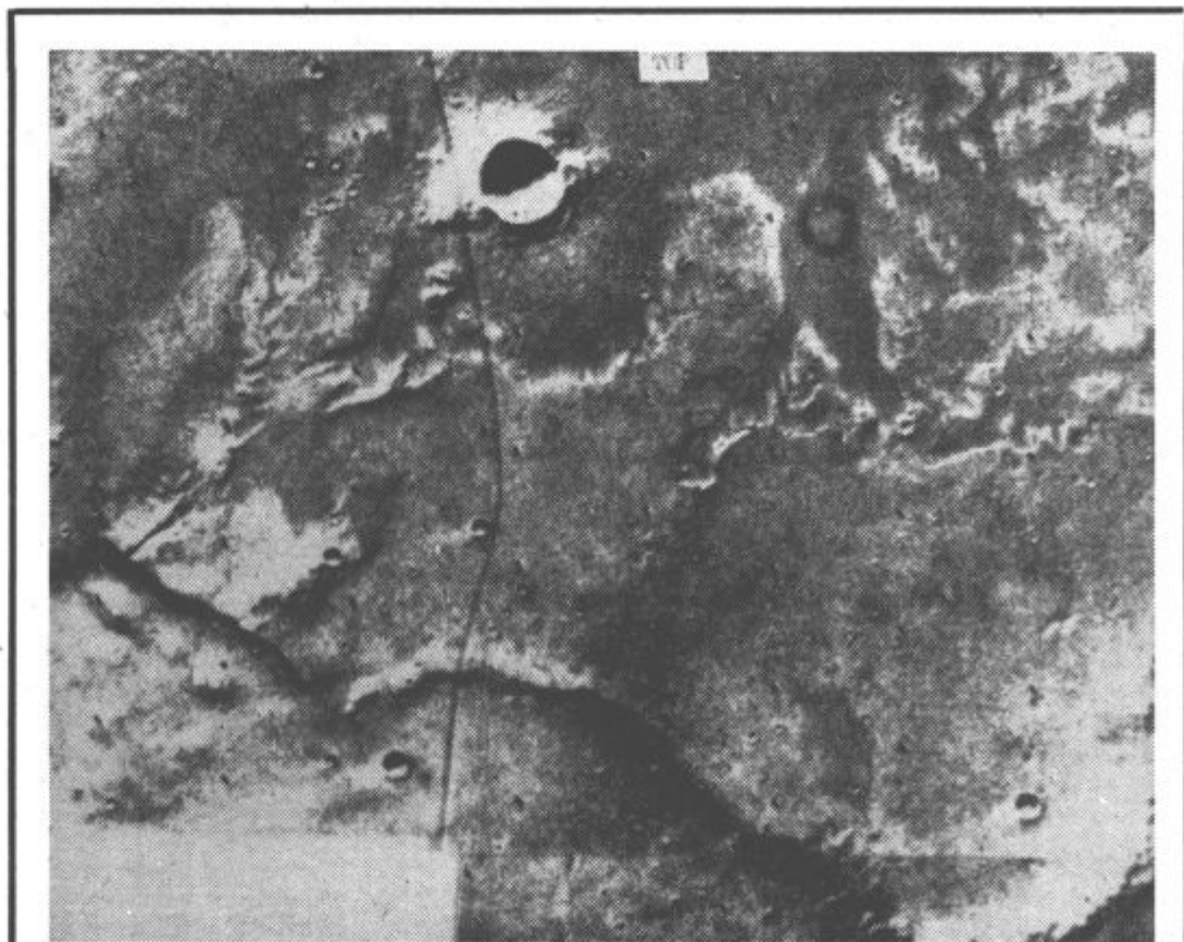
Mars znova in znova buri duhove znanstvenikom. Obstoj namreč možnost, da na Marsu je, ali je bila voda. Na sliki, ki jo je posnela medplanetarna sonda „Viking 1“ je namreč jasno vidno kako je voda oblikovala južni del planote (spodaj), to pa je povsem nova teorija o tem planetu.
