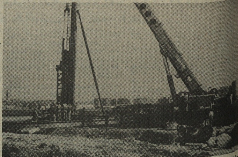
Za zabijanje pilotov smo si morali izposoditi 100 tonsko avtovigalo BTC iz Ljubljane, ki je največje v Sloveniji
