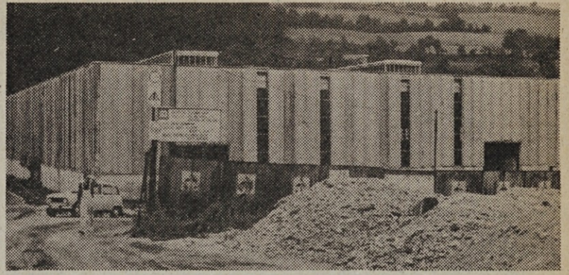
Nova jeklolivarna za Železarno Ravne je v zaključni fazi gradnje
