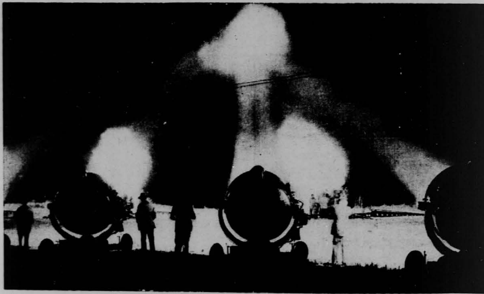
Velikanski žarkometi s premerom loče 60 palcev in z 800,000,000 sveč močno lučjo iščejo v artilerijski trdnjavi Monroe cilj, katerega vleče za seboj aeroplan, ki leti 6000 čevljev visoko. Ko artileristi zagledajo cilj, tedaj namerijo nanj 3-palčne protizračne topove. Ameriška armada ima na razpolago najmodernejši tip protiletalskih topov.
