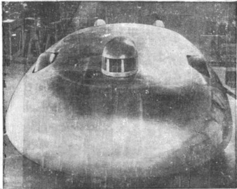
POŠASTI ZA DIRKANJE. S tem dirkalnim avtom namerava John Cobb na dirkalni progi v izsušenem slanem jezeru v državi Utah brzeti s hitrostjo nad 500 km/h in prekositi vse dosedanje avtomobilske hitrostne rekorde. Vozačev sedež je pod malim opazovalnim stolpičem, ki ga vidimo na vrhu jeklene pošasti
