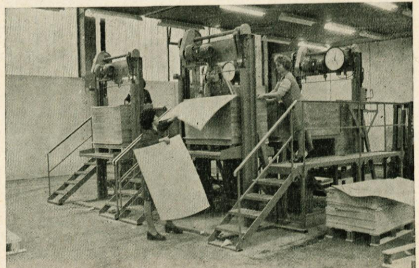
Priprava za embalaranje in tehtanje kartona
