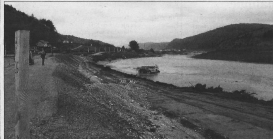
Izgradnja tesnjenega visokovodnega nasipa med potokoma Zdenski graben in Kolarjev graben - levi breg Save
