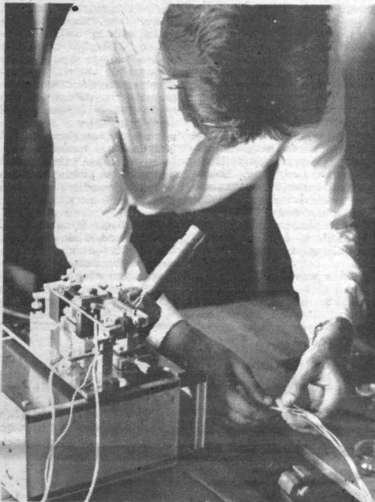
Na tekmovanju je bila prikazana tudi novost s področja kabelske tehnike – optični kable. Spajanje optičnega kabla so prikazali strokovnjaki Iskre, ki ga polaga na področju PTT podjetja Nova Gorica za potrebe Soških elektrarn. (Foto: Breda Malenšek)
