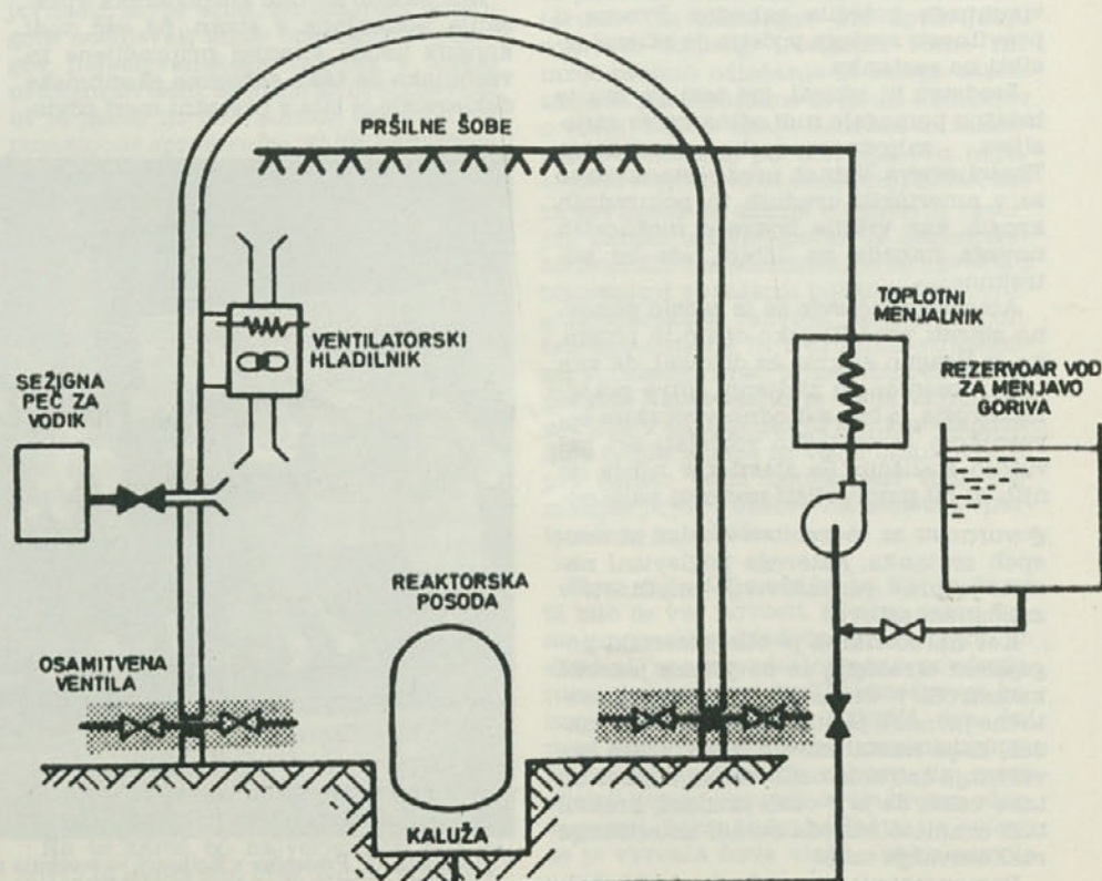
Skica zadrževalnega hrama v JE Krško in njegovih varovalnih sistemov
