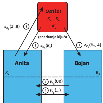
Slika 7. V prvem koraku Anita pošlje centru zašifriran zahtevek za pogovor z Bojanom. Center nato v drugem koraku generira ključ in ga pošlje obema. Bojanu tudi sporoči, kdo želi komunicirati z njim. Bojan v četrtem koraku pošlje sporočilo Aniti, da potrdi sprejetje ključa. Nato se začne komunikacija.
