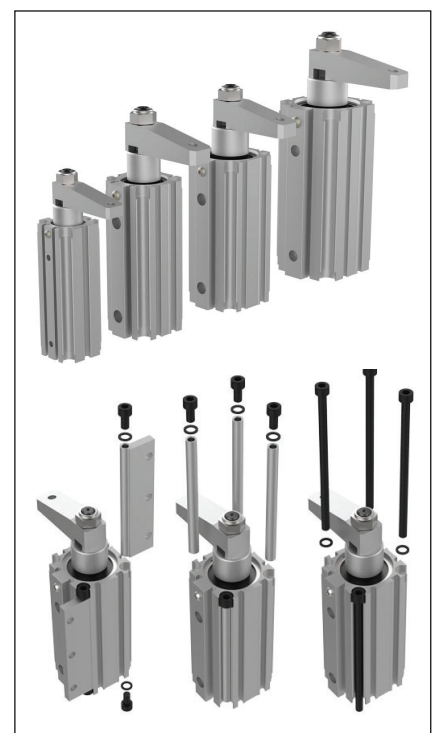
Prenovljena družina vpenjal serije 9500 (zgoraj) in možnosti pritrditve vpenjal serije 9500 (spodaj)
