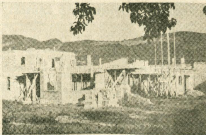
Kulturni dom v Moravčah raste. Po svojih razsežnostih zelo velika zgradba bo, ko bo dokončana, nudila streho vsem kulturnim in prosvetnim organizacijam v kraju, dvorana pa bo omogočila, da bodo Moravče končno dobile tudi svoj stalni kino. Upamo, da bo stavba pred jesenskim dežjem v celoti zaščitena in pokrita. Dom gradi Gradbeno podjetje Domžale.
