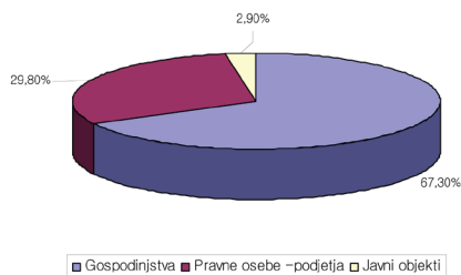
Slika 3: Delež porabe energije po vrsti porabnikov za ogrevno in tehnološko toploto
