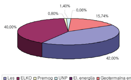
Slika 4: Delež porabe energije po vrsti energentov za ogrevno in tehnološko toploto v občini Veržej
