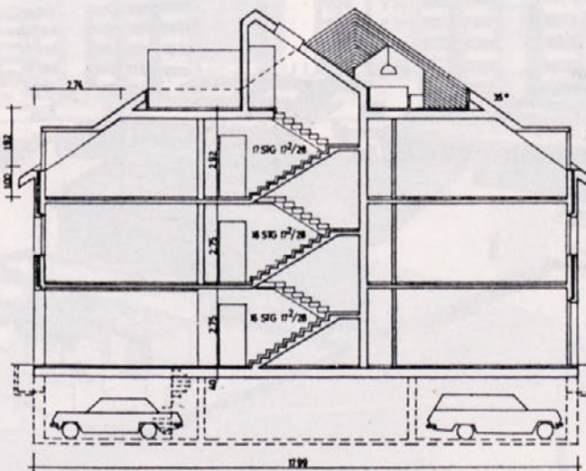
Prerez objekta
