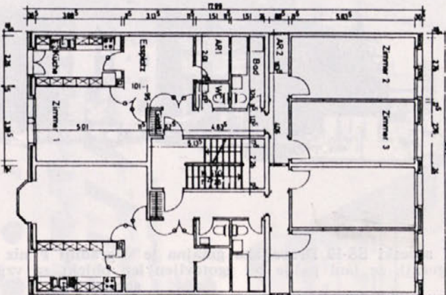
Tlorisna zasnova
