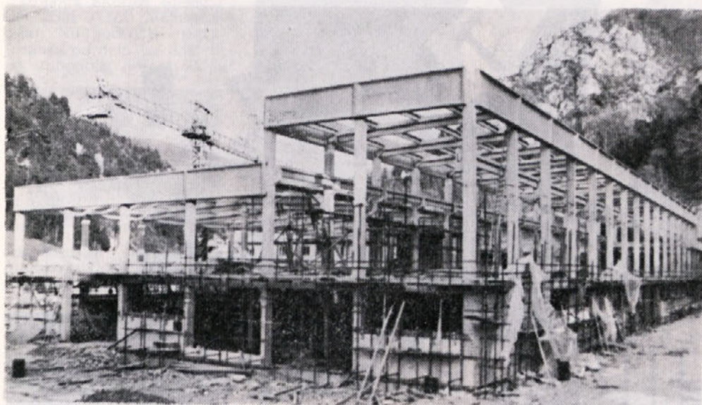
Leva slika prikazuje zmontirano Halo za papirni stroj v Radečah, na gornjem posnetku pa je dokončan viadukt nad železniško progo v Radečah
