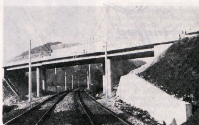
Leva slika prikazuje zmontirano Halo za papirni stroj v Radečah, na gornjem posnetku pa je dokončan viadukt nad železniško progo v Radečah
