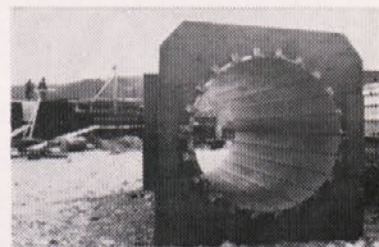
Kovinski opaž za okrogle stebre (od 90 do 200 cm premera)
