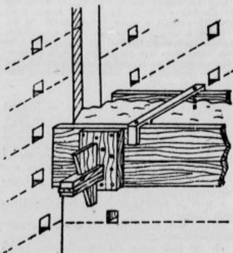
Sl. 10. Priključek vmesne stene na glavni zid.
