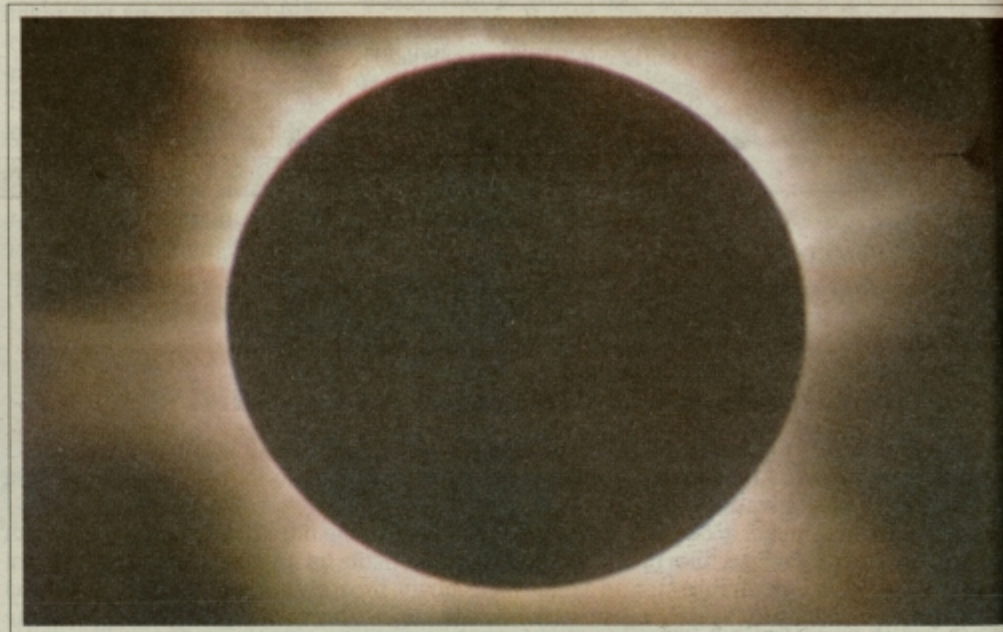
Sončeva korona, kot je vidna v času popolnega mrka.
