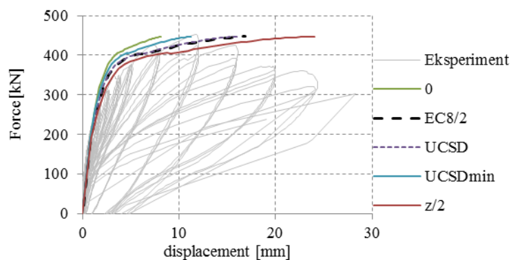
Slika 3.117: Primerjava med eksperimentalnimi rezultati in analitično histerezno ovojnico določeno z upoštevanjem različnih dolžin plastičnih členkov
