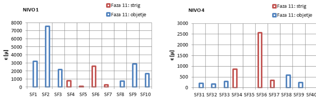
Slika 3.87: Največje dosežene deformacije na kompozitnih trakovih v fazi 11 na nivojih 1 in 4 Figure 3.87: Maximal strains at SGs on FRPs in phase 11 at levels 1 and 4
