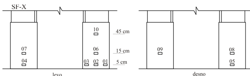
Slika 4.25: Položaj merilnih lističev na CFRP plašču
