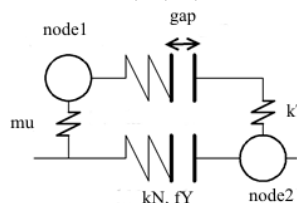
Slika E.1: Shema kontaktnega elementa – vzdolžna vzmet deluje kot stikalo za prečno vzmet Figure E.1: Element scheme - spring in normal direction acts like a switch for transverse direction
