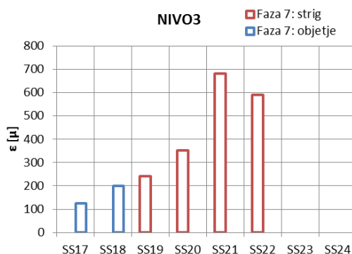
Slika 3.68: Največje dosežene deformacije v stremenih v fazi 7 na nivoju 3 (za položaj merilnih lističev glej načrt merskih mest - Slika 3.55)
