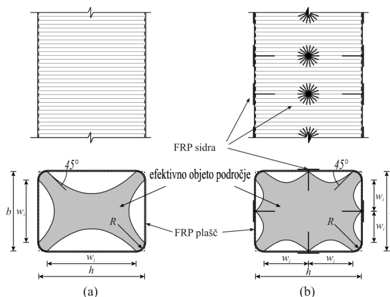
Slika 2.60: Možnosti za izboljšanje učinkovitosti objetja v pravokotnih stebrih z uporabo CFRP sider Figure 2.60: Possibilities for confinement effectiveness improvement in rectangular sections with the use of CFRP anchors
