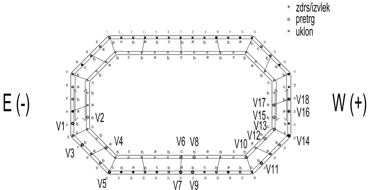
Slika 3.109: Tip porušitve zunanjih vzdolžnih palic
