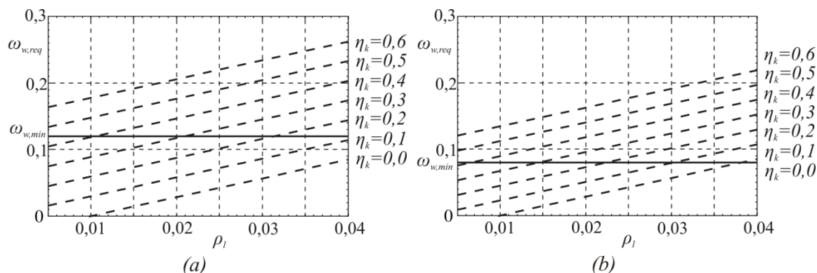
Slika 2.14: Mehanski delež objetja v odvisnosti od količine vzdolžne armature in nivoja osne sile za primer visoke duktilnosti (c) in primer srednje duktilnosti (b), kot ga zahteva EN1998-2 (CEN 2005c)
