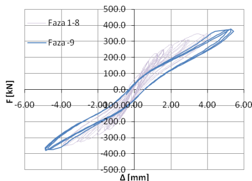
Slika 3.78: Odnos sila-pomik do vključno 9. faze Figure 3.78: Force-displacement relation until phase 9
