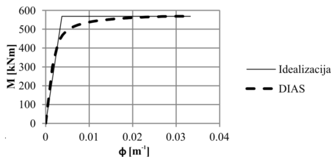
Slika 3.34: Elasto-plastična idealizacija krivulje moment-ukrivljenost za model NDŠS Figure 3.34: Elastic-plastic idealisation of moment-curvature relationship for specimen NDŠS
