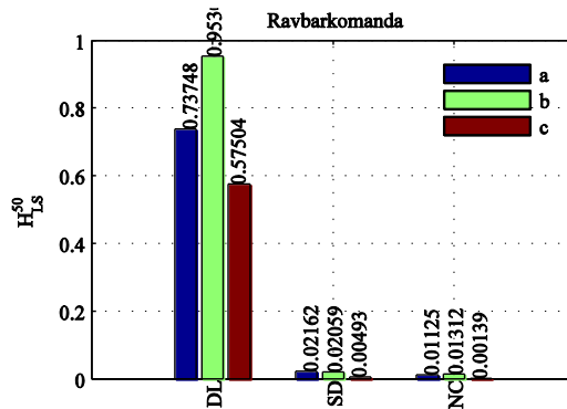
Slika 5.58: Verjetnosti prekoračitve izbranih mejnih stanj za daljši viadukt z različnimi kombinacijami fiksnih in drsnih ležišč
