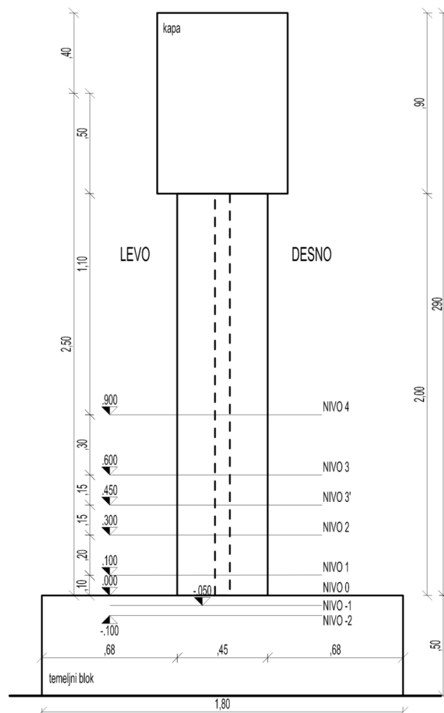
Slika 4.12: Višine nivojev merilnih lističev Figure 4.12: Strain gauge level heights
