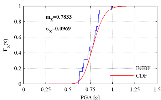
Slika 5.13: Primerjava empirične kumulativne funkcije porazdelitve PGA pri katerem pride do mejnega stanja pomembnih poškodb, t.i. krivulja ranljivosti (modra) in teoretične CDF (rdeča).
