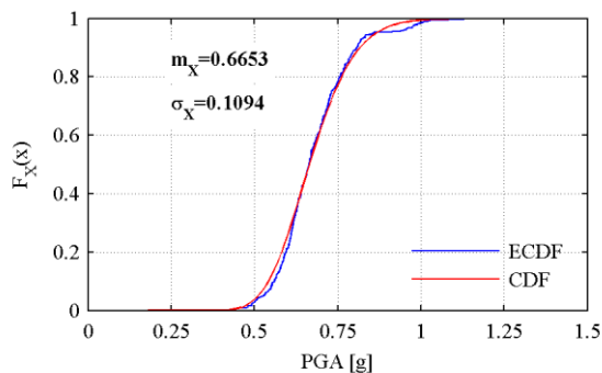
Slika 5.20: Primerjava empirične kumulativne funkcije porazdelitve (ECDF) (modra) in teoretične CDF (rdeča) PGA pri katerem pride do mejnega stanja pomembnih poškodb v primeru LHS
