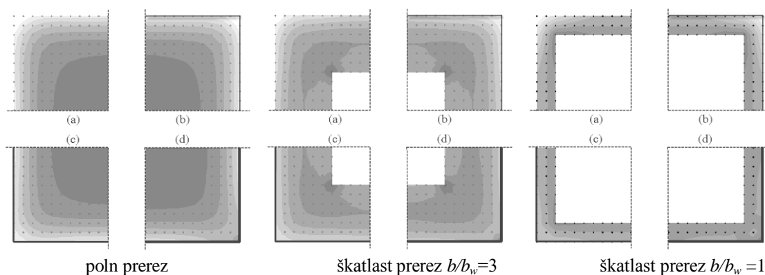
Slika 3.121: Napetosti v prerezu v odvisnosti od količine objetja: (a) brez objetja; (b) ena plast; (c) 4 plasti in (d) 8 plasti ter od oblike prereza
