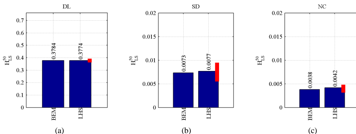
Slika 5.39: Primerjava tveganja za presežek izbranih mejnih stanj za BEM in LHS (z rdečo je označeno območje \pm\sigma )
