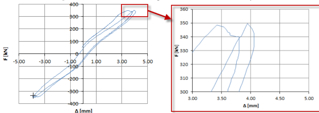
Slika 3.77: Padec sile pri maksimalnem doseženem pomiku cikla v fazi 8 Figure 3.77: Force drop at maximum cycle displacement in phase 8
