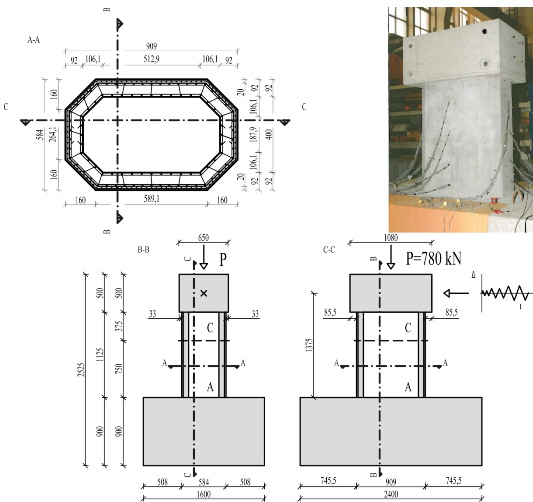
Slika 3.44: Geometrija modela stebra UKŠS-BPL.
