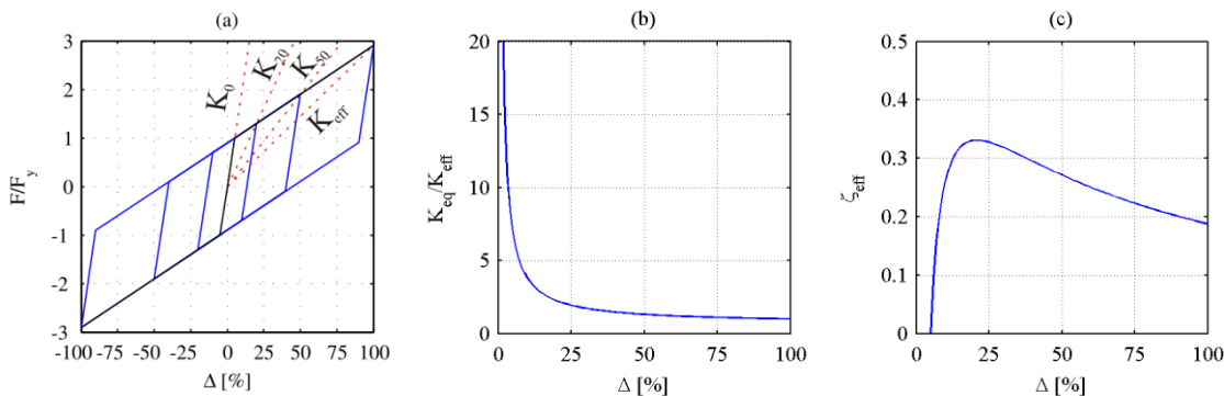
Slika 2.73: Idealizirana zveza med silami (a), ekvivalentno togostjo (b) in ekvivalentnim dušenjem (c) v odvisnosti od pomika za elastomerna ležišča
