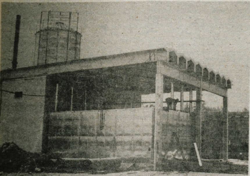
Nova sušilnica LIP-a v Mojstrani — Pri temeljni organizaciji LIP Mojstrana gradijo novo polavtomatsko sušilnico za les, z zmogljivostjo 36 kubičnih metrov v vsaki izmed dveh komor. Uporabljali jo bodo za sušenje trdih in mehkih lesov, avtomatske naprave pa so iz uvoza. Vrednost naložbe je 100 milijonov dinarjev, za mojstranski mojstranski LIP pa je precejšnja pridobitev, saj bodo lahko povečali svoj kvaliteten proizvodni program. Zdj izdelujejo vhodna in garažna vrata, z novo sušilnico pa bodo proizvodni program obogatili za nove stolice, ki jih bodo izvažali. — D. Sedej — Foto: F. Perdan
