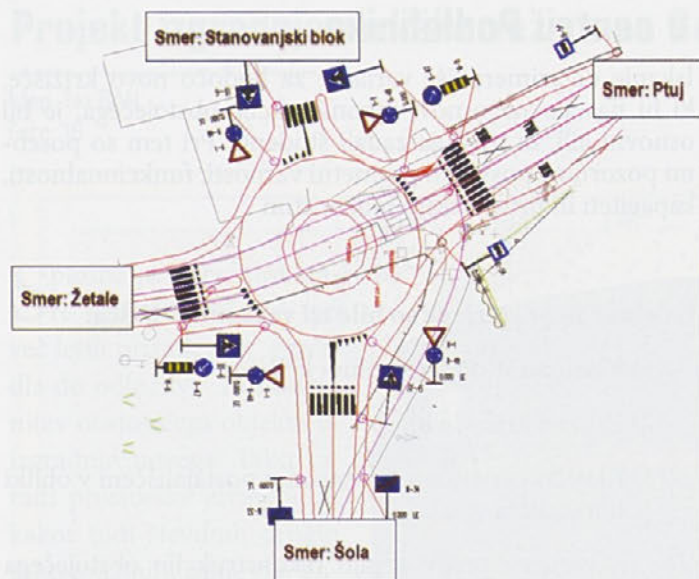
2 Varianta – Klasično krožno križišče
