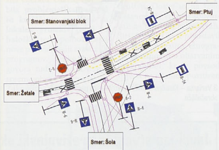
1 Varianta – Klasično štirikrako »plus« križišče
