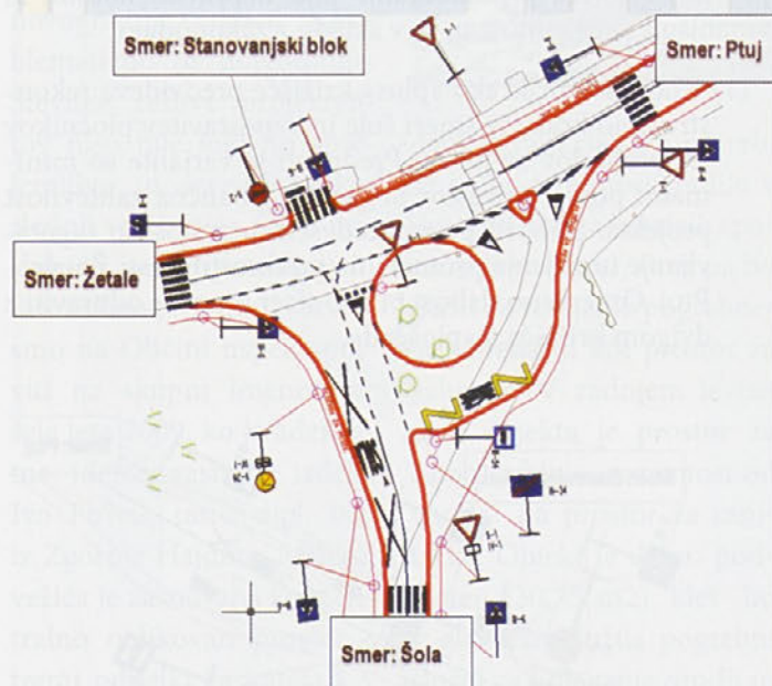
3 Varianta – Klasično križišče z avtobusnim postajališčem v obliki obračališča
