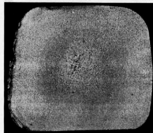
Sl. 24 — medkristalne razpoke v jeklu Č 4171
