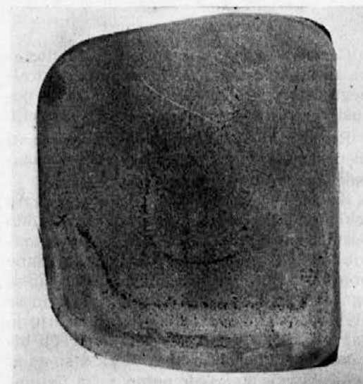
Sl. 22 — vključki v jeklu (delno zavihanje skorje pri litju)
