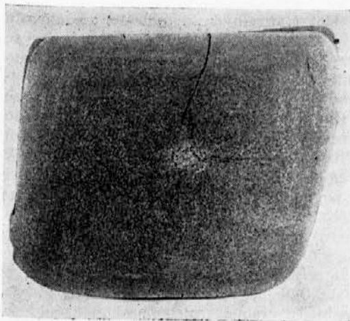
Sl. 25 — medkristalne razpoke v jeklu Č 4570
