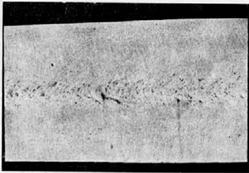
Sl. 19 — centralna poroznost v ingotu (vzdolžni prerez)
