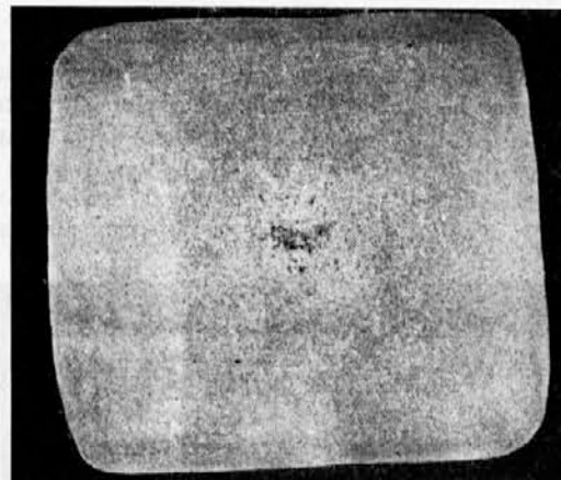
Sl. 17 — ostanek lunkerja v gredici
