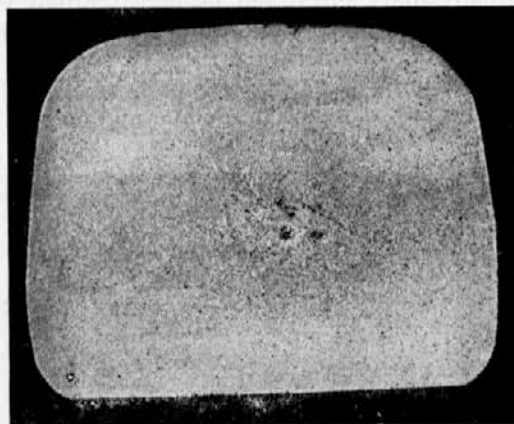
Sl. 20 — poroznost po celem preseku s centralno poroznostjo v sredini
