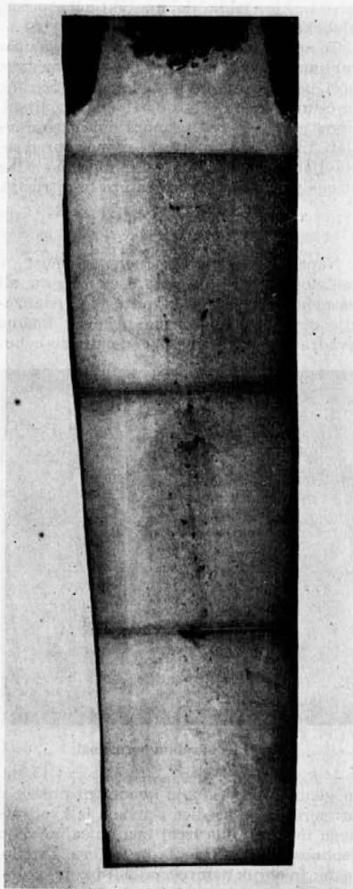
Sl. 16 — lepo izoblikovani lunker v glavi ingota (vzdolžni prerez) pri uporabi eksotermne kape
