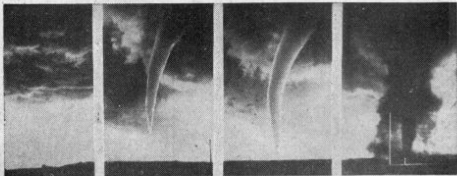
Od leve proti desni: preteči tornado neposredno pred izbruhom; začetek tornada; skoraj do zemlje segajoči lijak in tornado je dosegel zemljo
