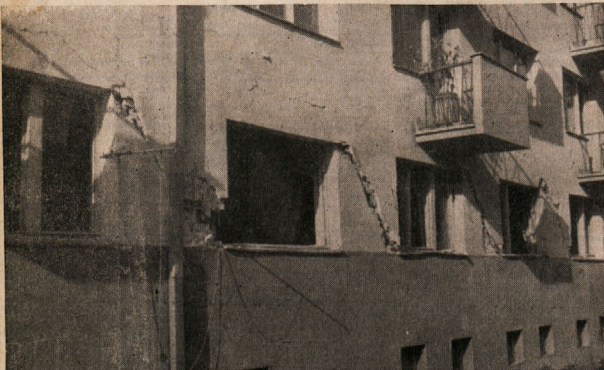
Najbolj karakteristične razpoke so se pojavljale v pritličjih objektov, ki so popolnoma potrdile teorijo o vplivu horizontalnih sil na konstrukcije
