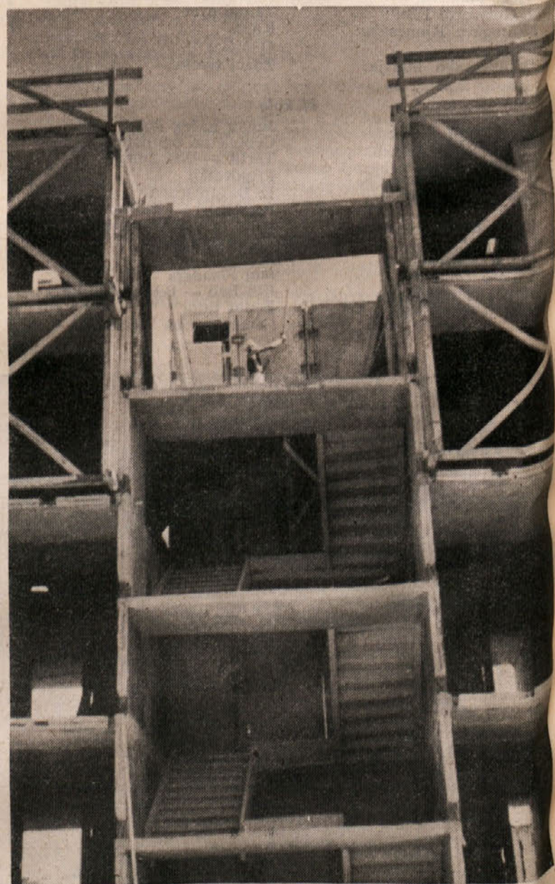
V enem tednu je 45-stanovanjska hiša na Otoku II. že imela »smreko«. Vse stanovanjske enote so enake, velikost stanovanja določa le različno število enot.
