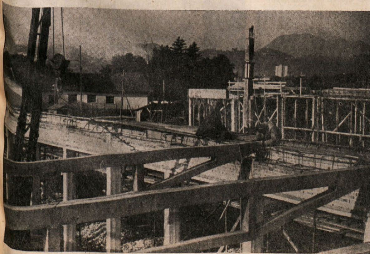
Objekt garaže na klavnici ima ostreže izvedeno iz montažnih predalčnih nosilcev in durisol plošč
