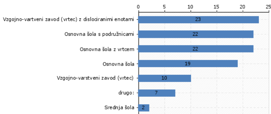
Slika 1: Struktura vzorca
