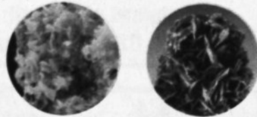
Autonit, nahajališče Bois Noirs, Francija Torbernit, nahajališče Bois Noirs, Francija
