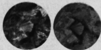
Metaautonit, pod UV svetlobo, nahajališče Novy Foitov, Češka
