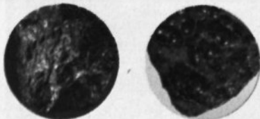
U-smola, nahajališče Jachimov, Češka Uraninit, nahajališče Jachimov, Češka
