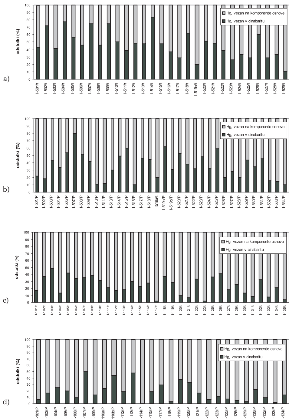
Slika 3. Razmerje med živim srebrom, vezanim v cinabaritu in vezanim na komponente osnove v vzorcih:
