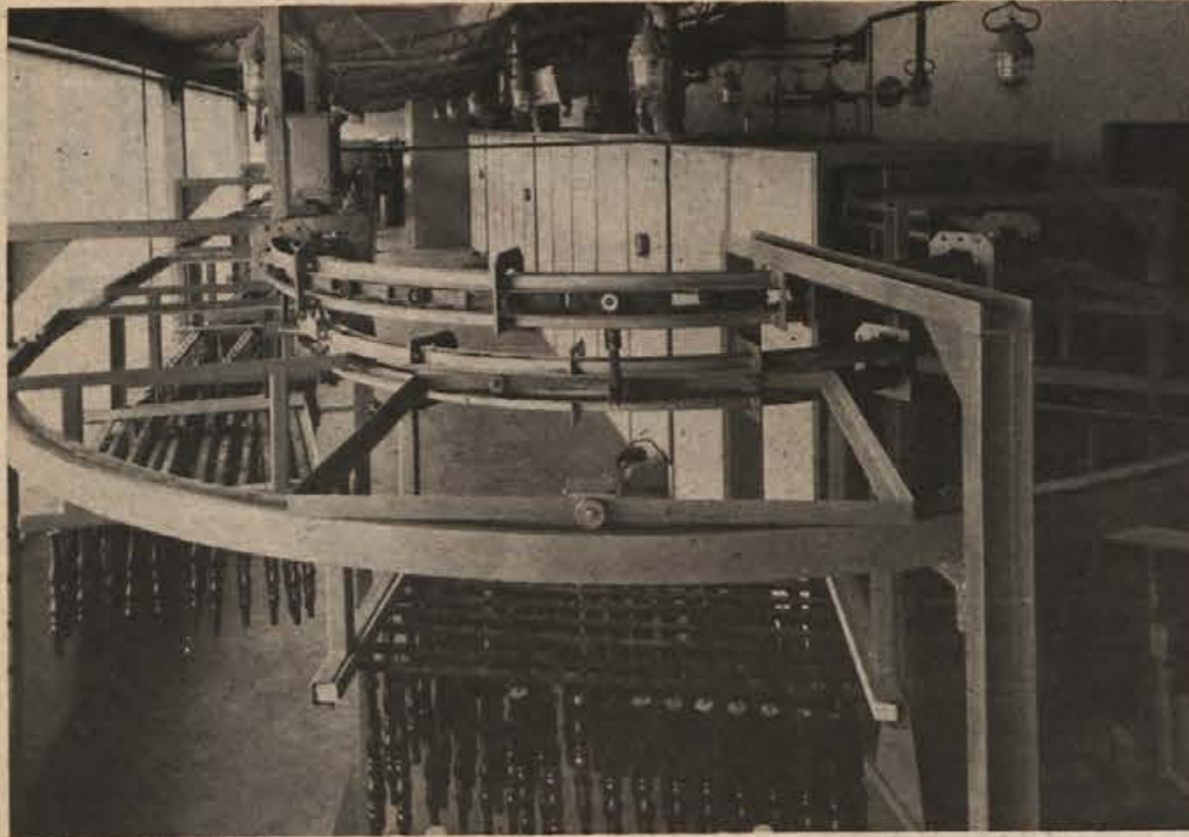
Lakirna linija za lesno industrijo v tovarni LIP RADOMLJE, ki jo je projektiral in izdelal SOP Krško.
