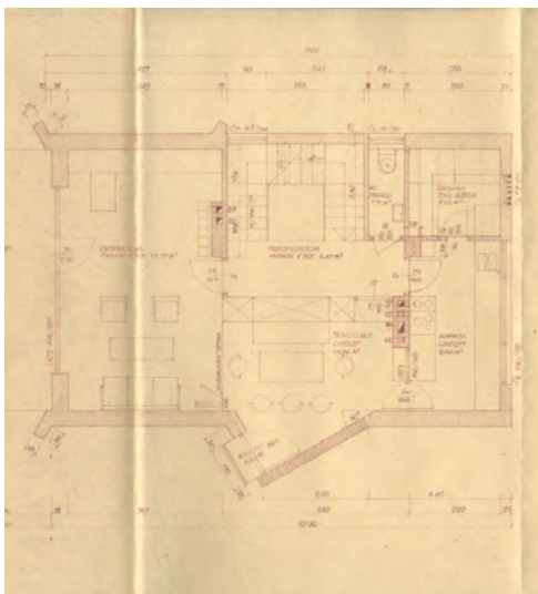
Načrt za enostanovanjsko hišo Dušana Muleja, tloris pritličja, 1962 (ZAL, VRH 18).
