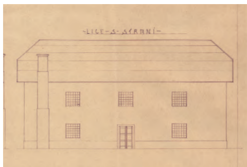
Načrt za skladišče k Pišlerjevi destilarni, stranski ris, 1943 (ZAL, VRH 2).
