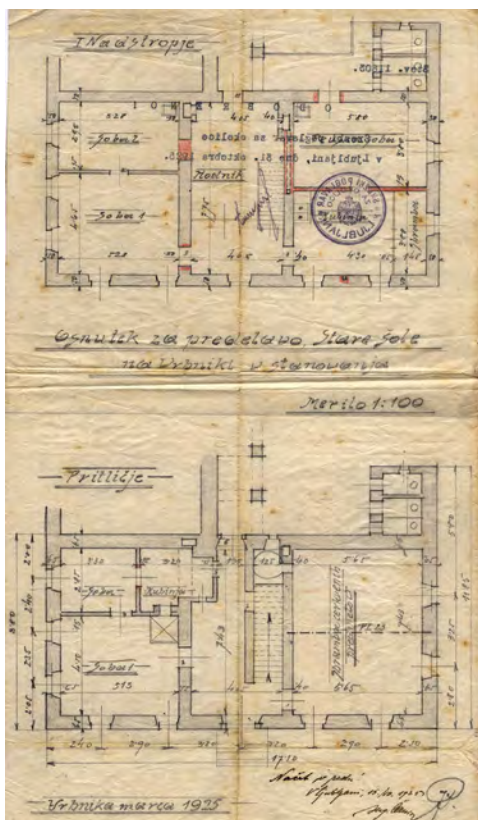
Načrt za prenovo stare šole, 1925 (NŠAL, ŽA Vrhnika).
