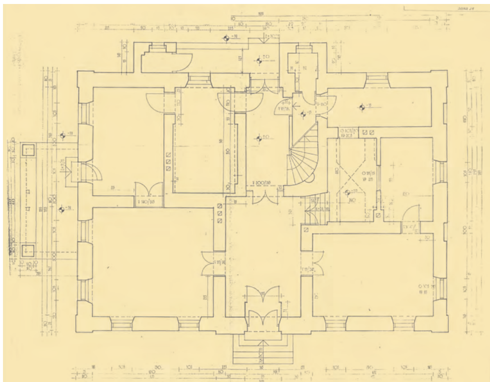
Floris pritličja.
