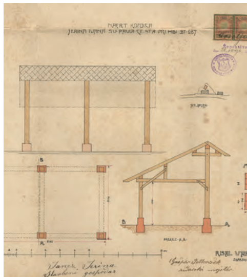
Načrt za gradnjo kozolca Janeza Jerine, 1908 (ZAL, VRH 2).
