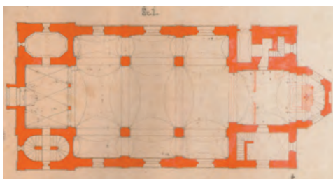
Floris župnijske cerkve sv. Pavla, s. d. (M. Ambrožič, Župnijska cerkev spreobrnjenja sv. Pavla na Vrhniki).
