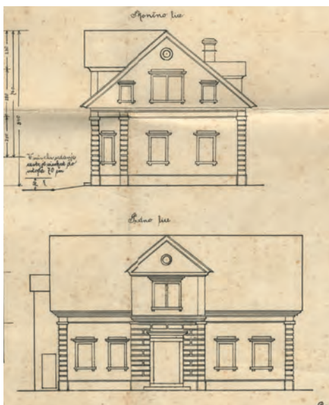
Načrt za predelavo hiše Ignacija Stržinarja, 1910 (ZAL, VRH 2).
