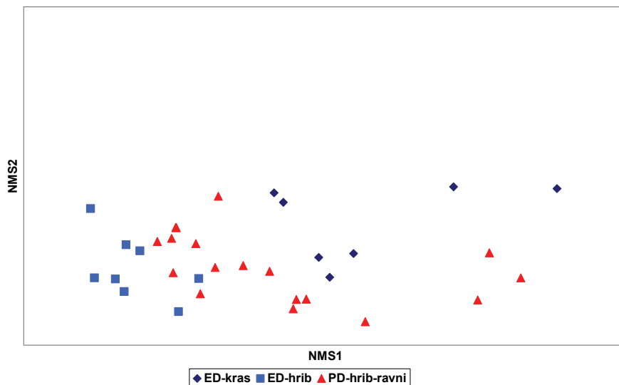
Slika 6. Ordinajski diagram nemetričnega multidimenzionalnega skaliranja vzorčnih mest na podlagi bentoških nevretenčarjev. Simboli označujejo bioregije: ED-kras – Dinarski kras, ED-hrib – Dinarska hribovja, PD-hrib-ravni – Preddinarska hribovja in ravnine. Faktor stresa (stress) = 0,12.
