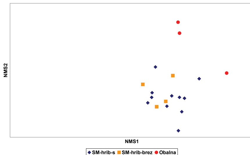
Slika 7. Ordinajski diagram nemetričnega multidimenzionalnega skaliranja vzorčnih mest na podlagi bentoških nevretenčarjev. Simboli označujejo bioregije: SM-hrib-s – Submediteranska hribovja s površinskim odtokom, SM-hrib-brez – Submediteranska hribovja brez površinskega odtoka, Obalna – Obalna gričevja. Faktor stresa (stress) = 0,12.
