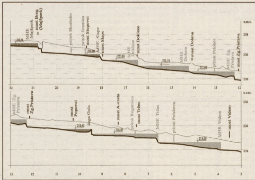
Vzdolžni profil Dravinje od tretjega do 22 km s predvidenimi zaježitvami malih hidroelektrarn.
