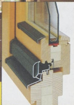
Energijsko varčno leseno okno z izolacijo
