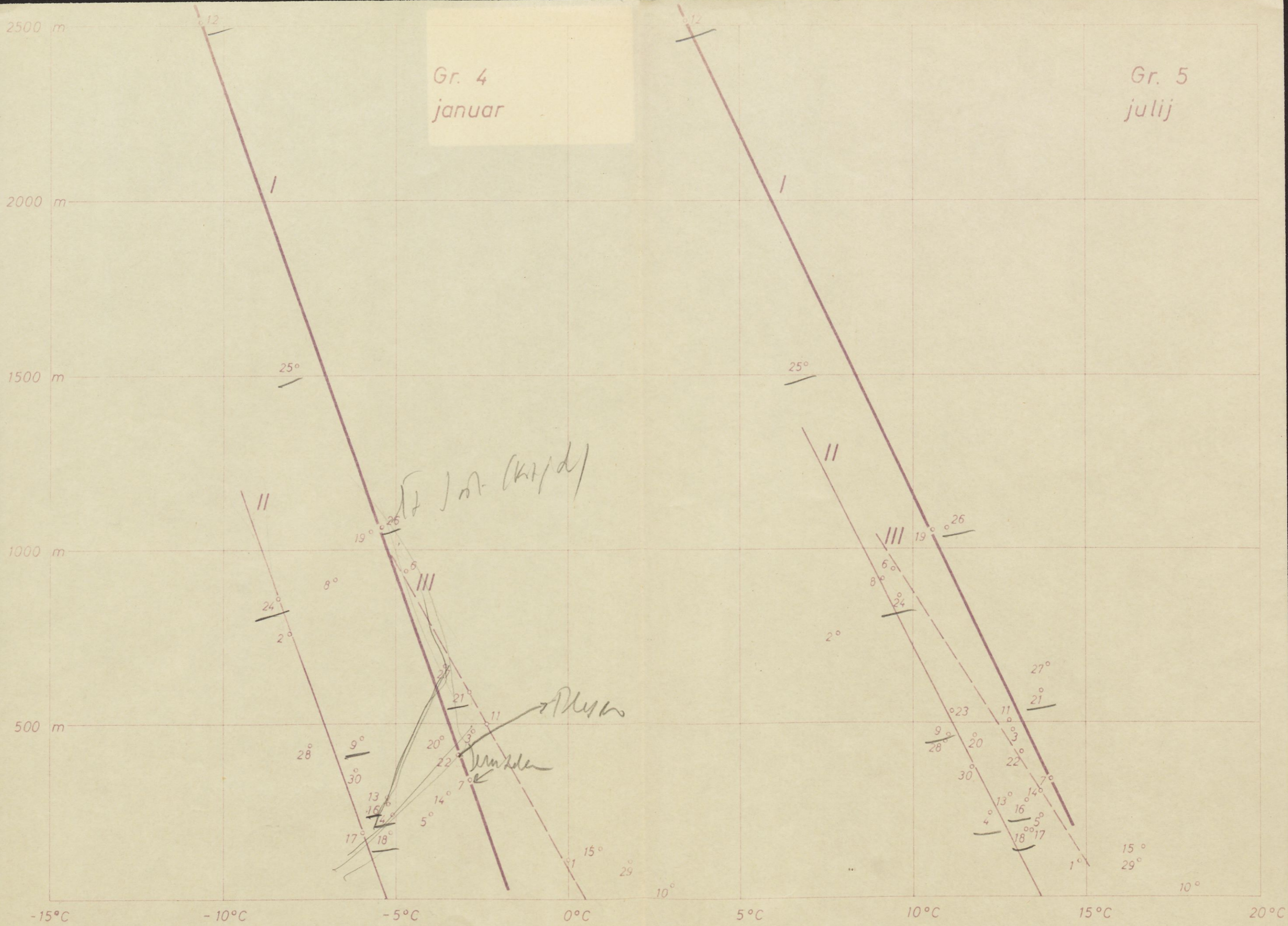
RAZPOREDBA SREDNJIH MINIMALNIH TEMPERATUR 1931-1960
