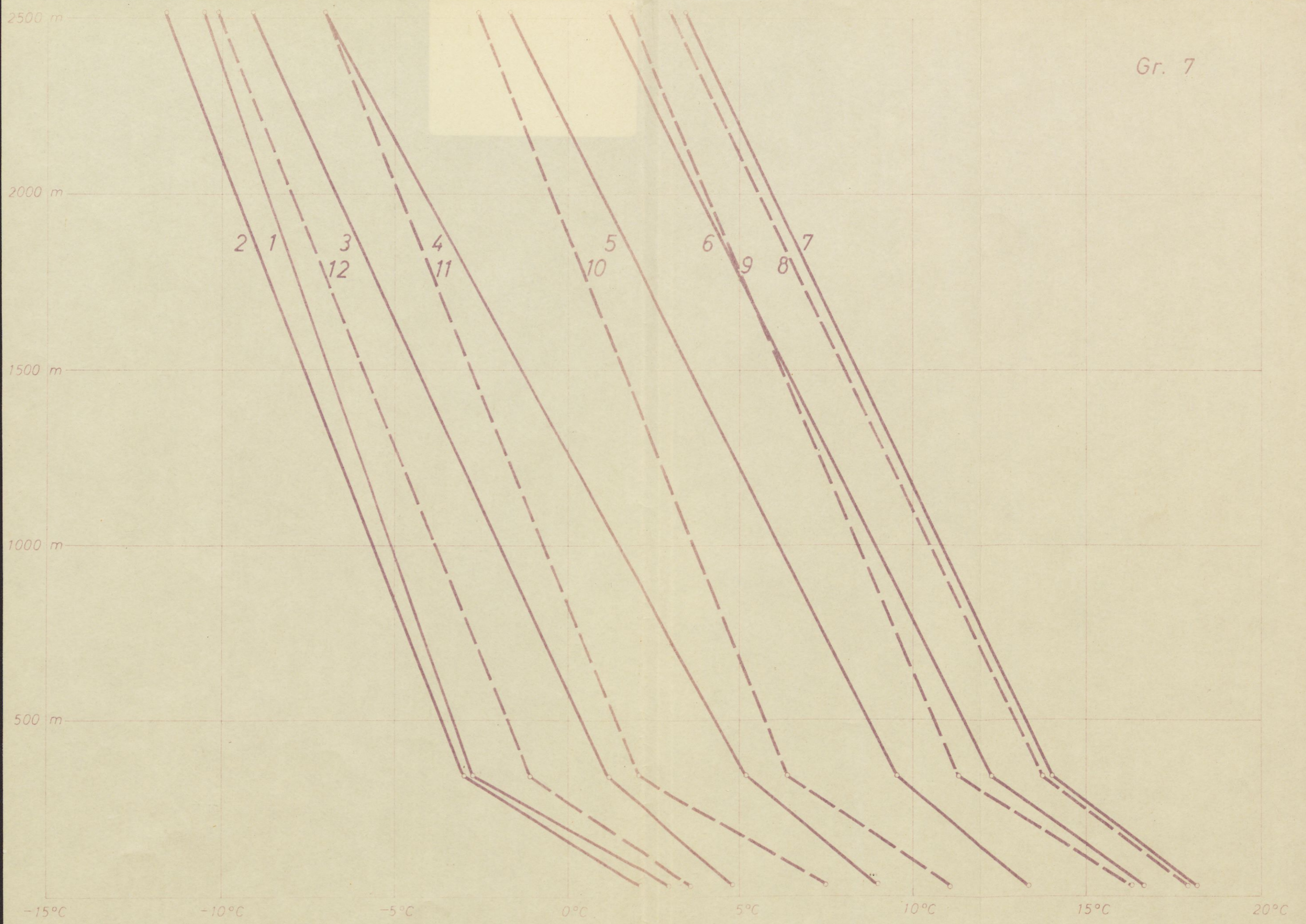
VERTIKALNI GRADIENTI SREDNJIH MESEČNIH MINIMALNIH TEMPERATUR 1931-1960
