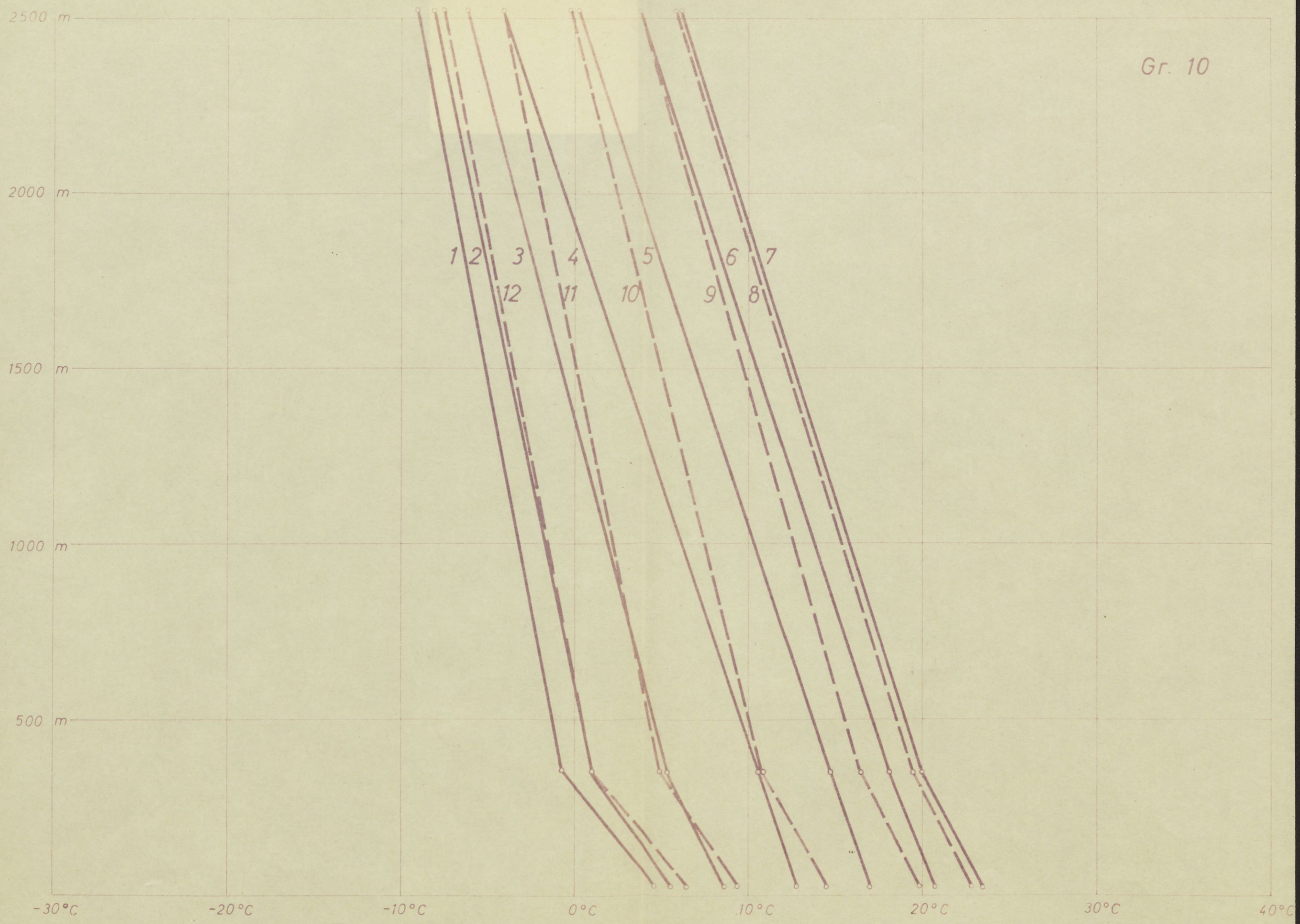
VERTIKALNI GRADIENTI SREDNJIH MESEČNIH TEMPERATUR 1931-1960
