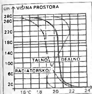
Temperaturni vertikalni profil v prostoru pri različnih ogrevilih
