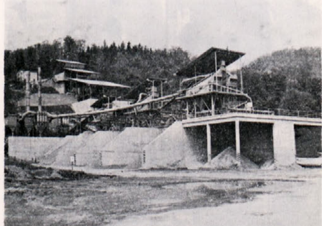
Kamnolom Zagaj pri Rogaški Slatini — deponijski boksi klasirnice se bodo po opustitvi kamnoloma uporabili v druge namene.
