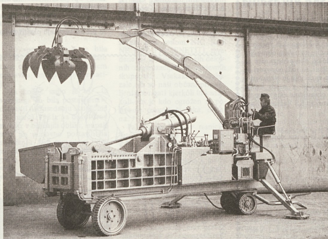
Stiskalnica za kovine S-125 z nakladalcem RN-3 a. Večji del proizvodnje je namenjen izvozu v Sovjetsko zvezo.
