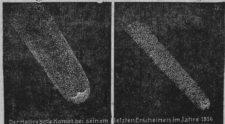
Der Halley'sche Komet bei seinem letzten Erscheinen im Jahre 1836
